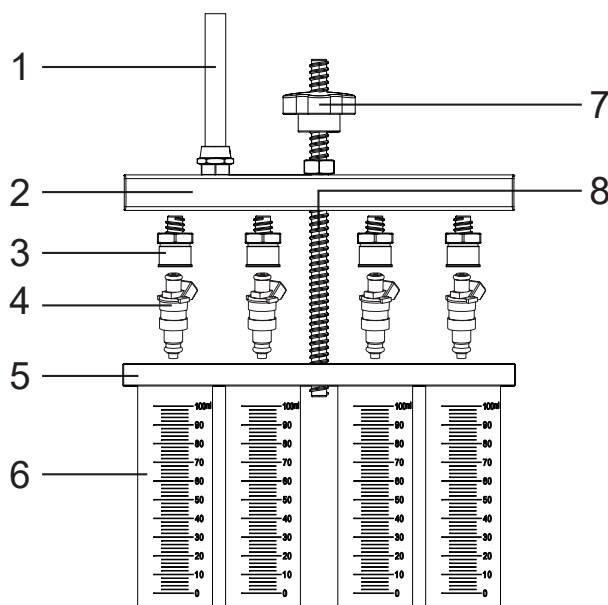
Diagramm zur Installation des oberen Kraftstoffinjektors
